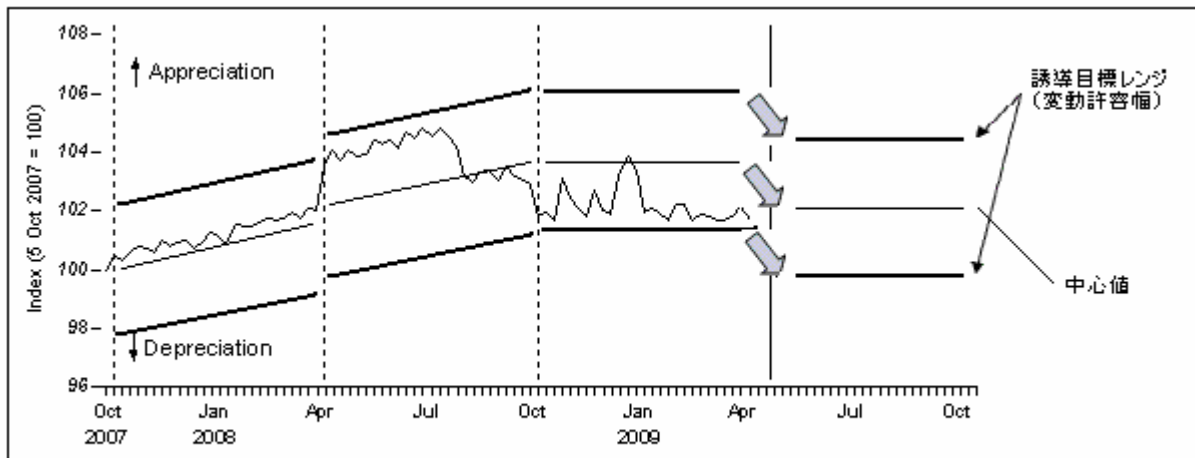
S$NEER 推移
