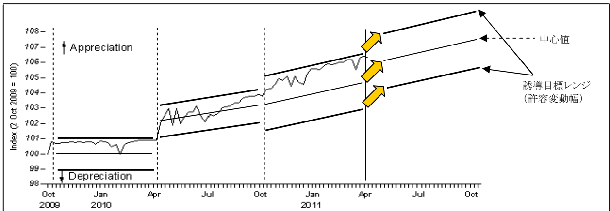
S$NEER 推移
